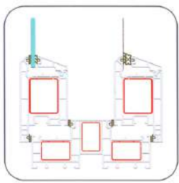
Twin Sash Door
